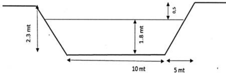
CORTE FRONTAL
